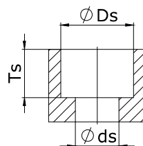
Senkbohrung
